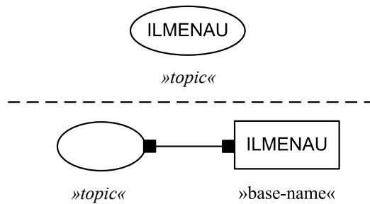
Fig. 4. Topic names shortcut
